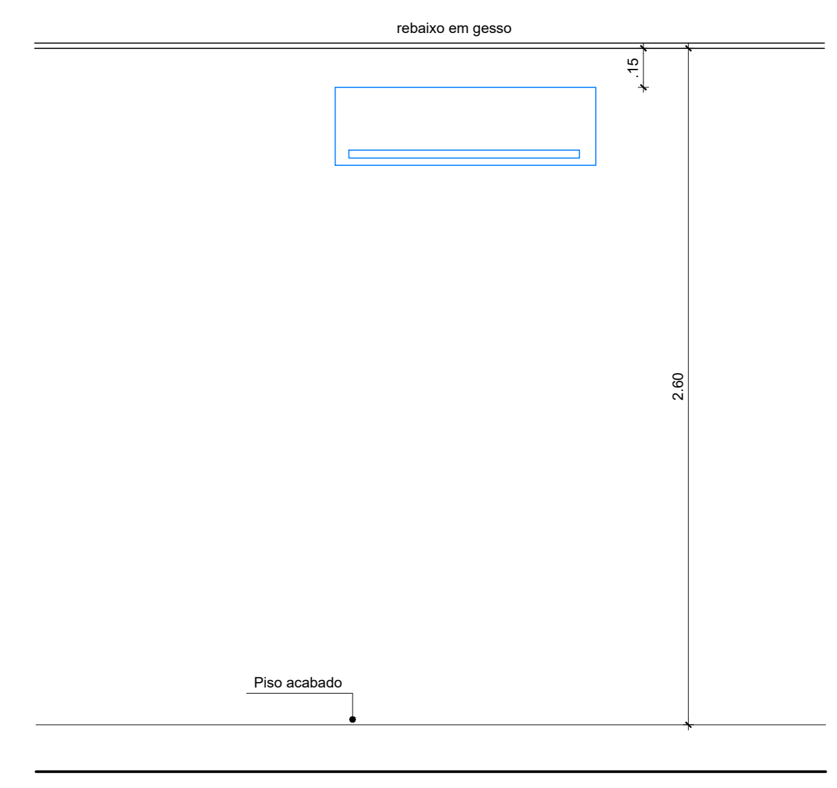
VISTA REFERÊNCIA ALTURA AR CONDICIONADO ESC: 1/20
